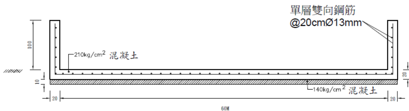
A-A池體剖面示意圖
